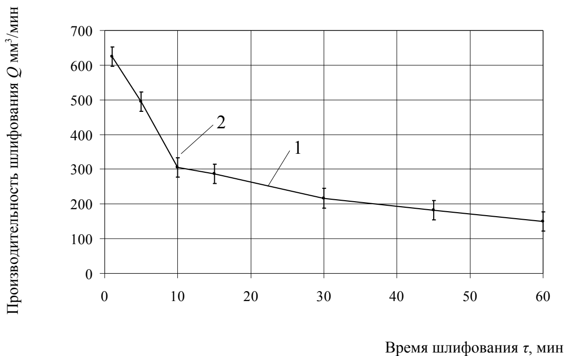
Рис. 3. Изменение текущей лимитированной режущей способности круга 1А1 250×76×15×5 АС6-100/80-4-М2-01 при шлифовании комбинированного образца «сталь 45- твердый сплав ВК8»: 1 – экспериментальные данные; 2 – регрессионная зависимость
