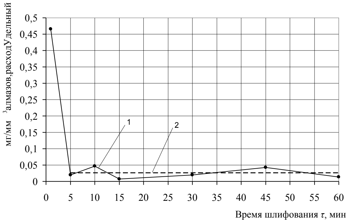
Рис. 4. Удельный расход алмазов в процессе шлифования комбинированного образца «сталь 45 – твердый сплав ВК8» кругом 1А1 250×76×15×5 АС6-100/80-4-М2-01: 1 – экспериментальные данные; 2 – средняя величина расхода алмазов
